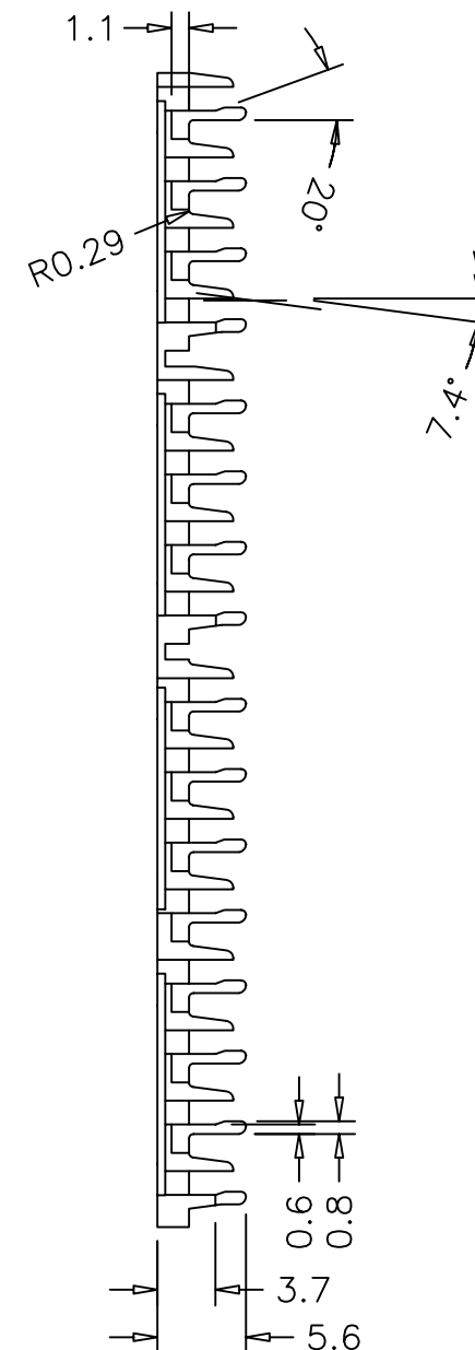
SECTION A-A
